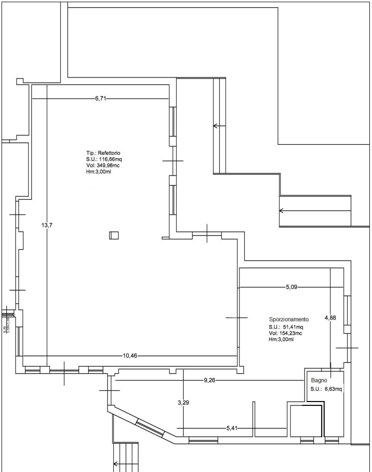
PLANIMETRIA ISTITUTO T. SILVESTRI VIA DEI LECCI
